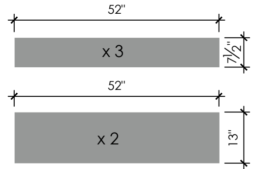
FILLER PANELS**
